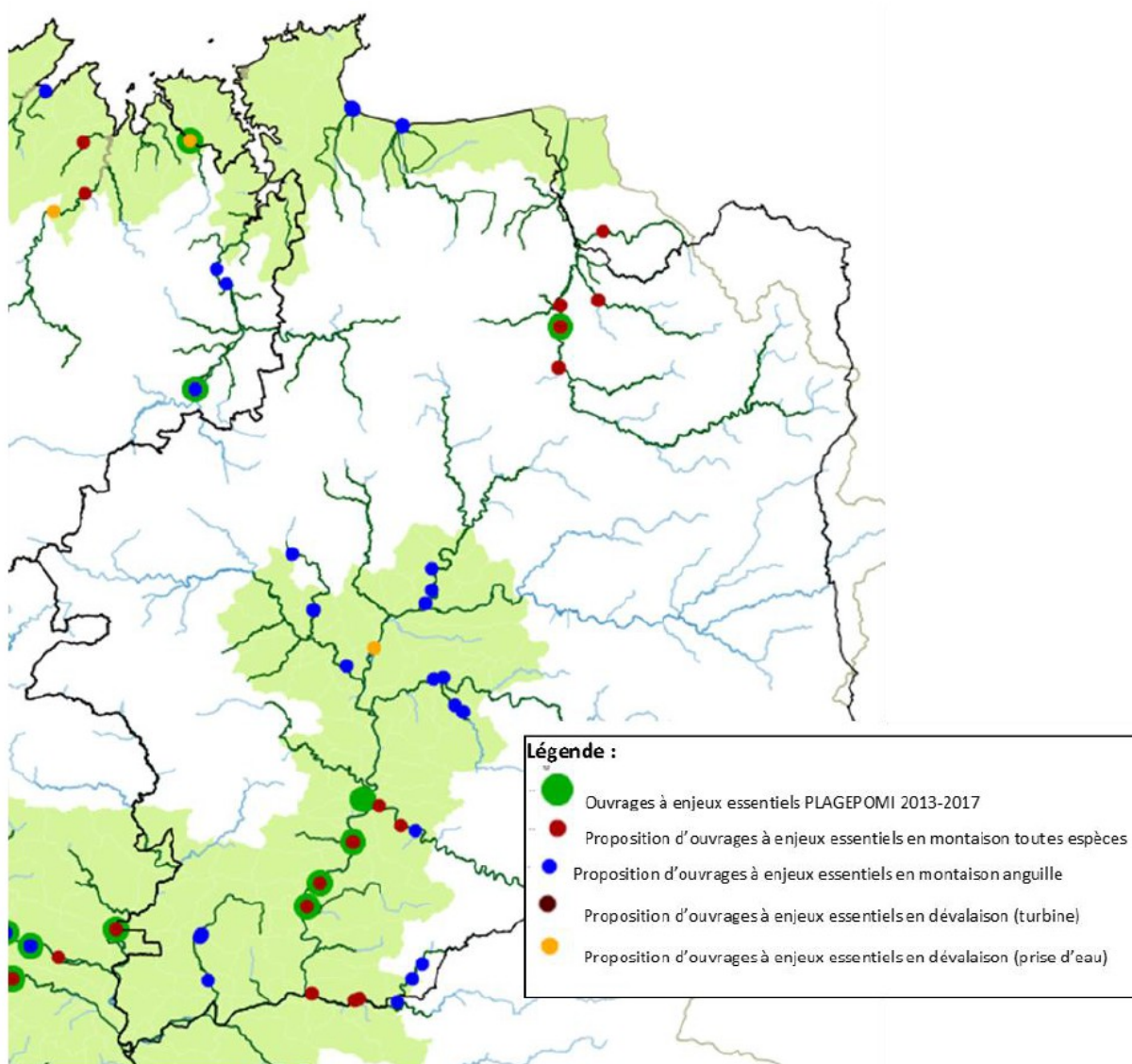
Figure 5 : Proposition d'ouvrages à enjeux essentiels PLAGEPOMI 2018-2023 – MONTAISON et DEVALAISON dans le département de l'Ille-et-Vilaine
