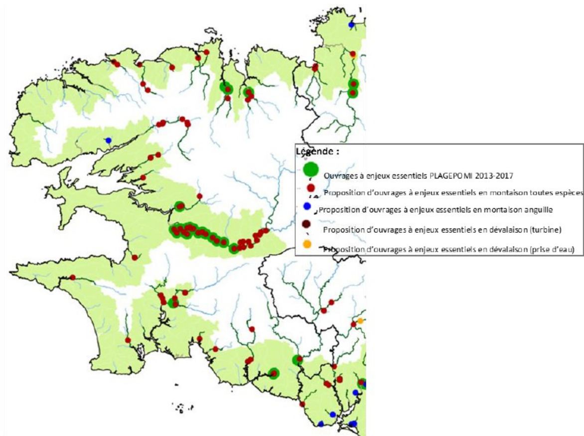
Figure 4 : Proposition d'ouvrages à enjeu essentiel PLAGEPOMI 2018-2023 – MONTAISON et DEVALAISON dans le département du Finistère
