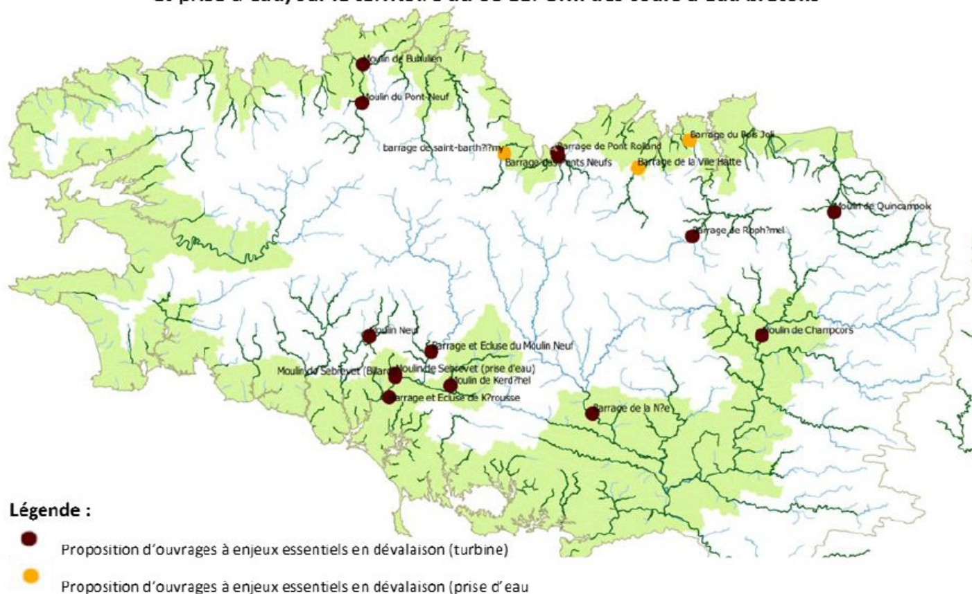
Figure 2 : Proposition d'ouvrages à enjeu essentiel PLAGEPOMI 2018-2023 – DEVALAISON (turbines et prise d'eau) sur le territoire du COGEPOMI des cours d'eau bretons
