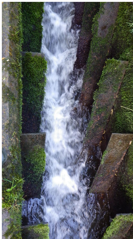
Figure 5 : Passe à ralentisseur (crédit photo : G. GERMIS – Bretagne Grands Migrateurs)
