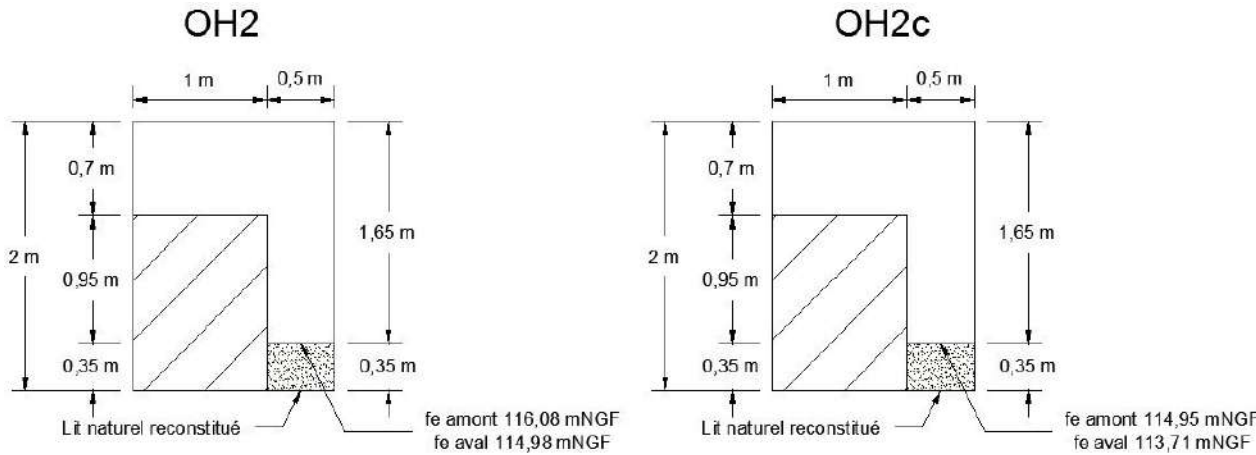
Figure 8 : Thalweg 2 - ouvrages projet
