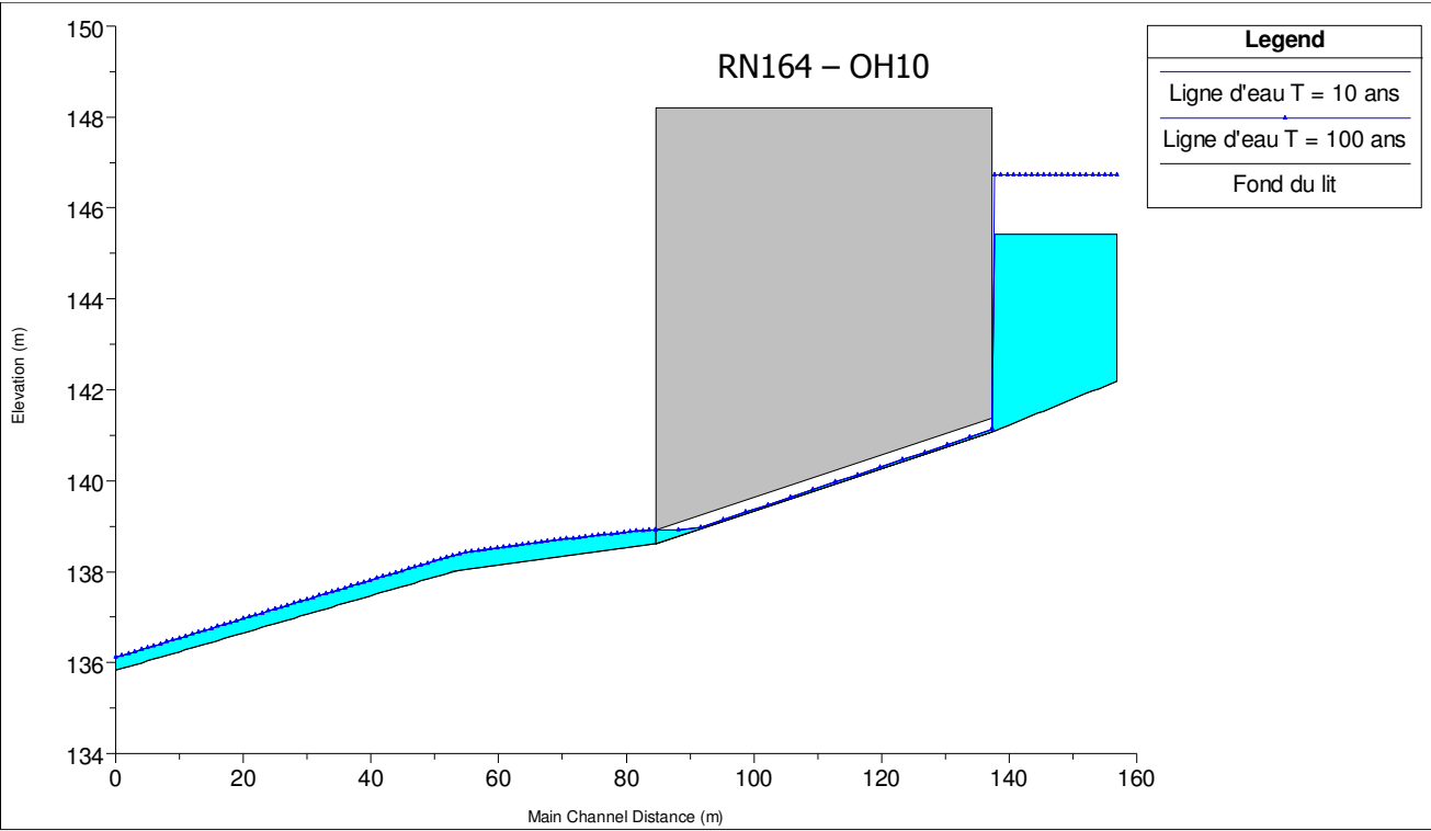
Figure 22 : Thalweg 10- Lignes d'eau au droit de l'ouvrage - Etat initial
