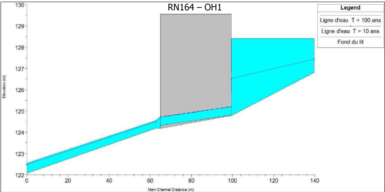
Figure 2 : Thalweg 1 - Lignes d'eau au droit de l'ouvrage - Etat initial
