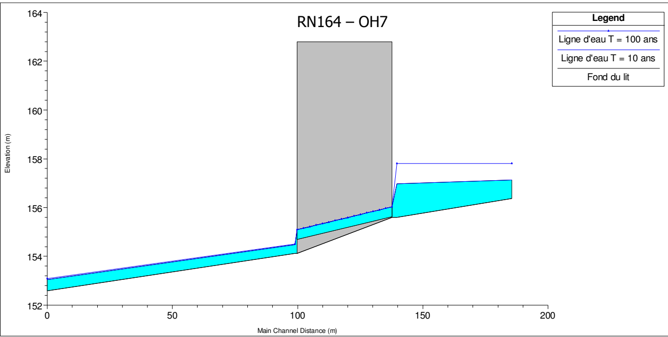
Figure 19 : Thalweg 7- Lignes d'eau au droit de l'ouvrage - Etat initial
