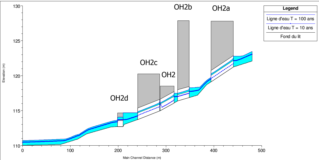
Figure 9 : Thalweg 2 - Lignes d'eau au droit de l'ouvrage - Etat projet
