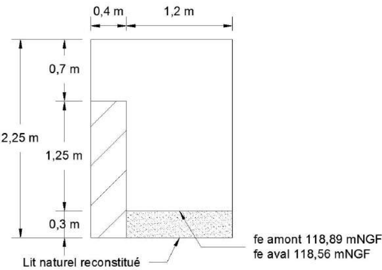
Figure 14 : Thalweg 5 - Ouvrage projet
