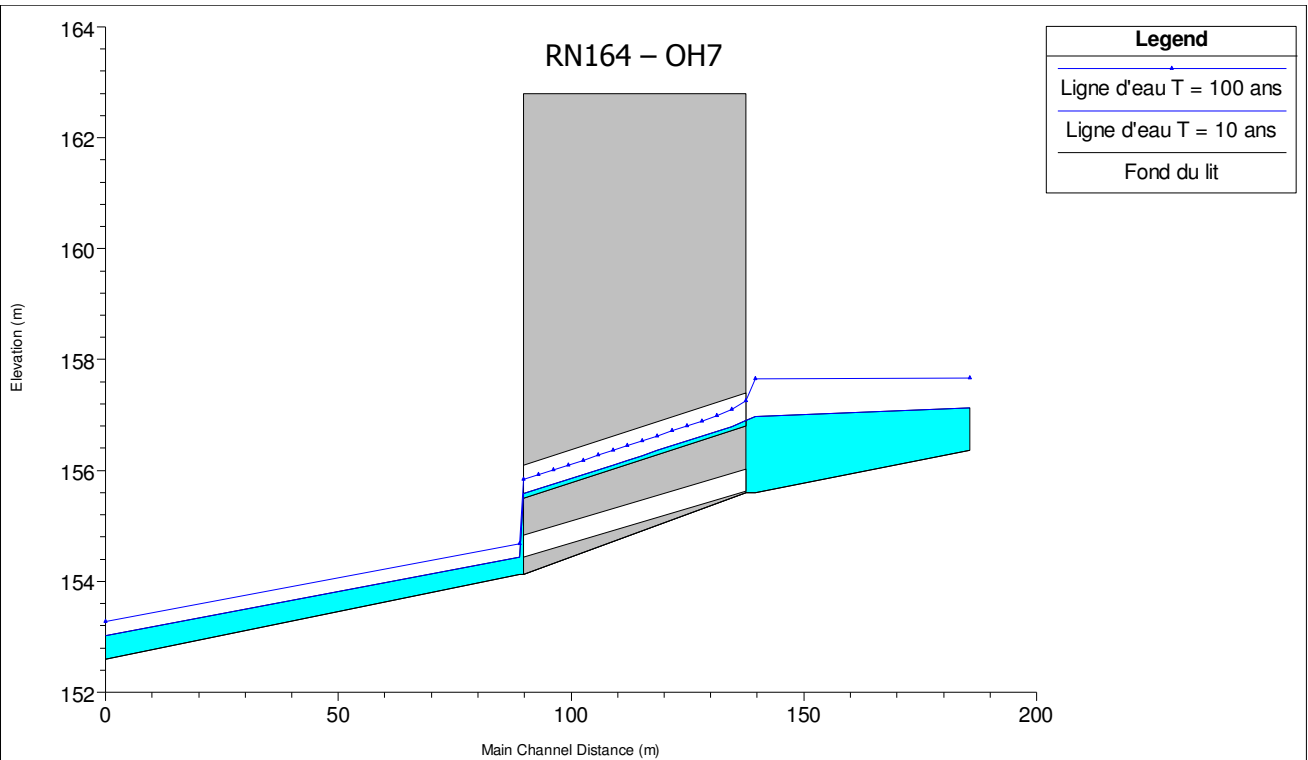
Figure 20 : Thalweg 7- Lignes d'eau au droit de l'ouvrage - Etat projet
