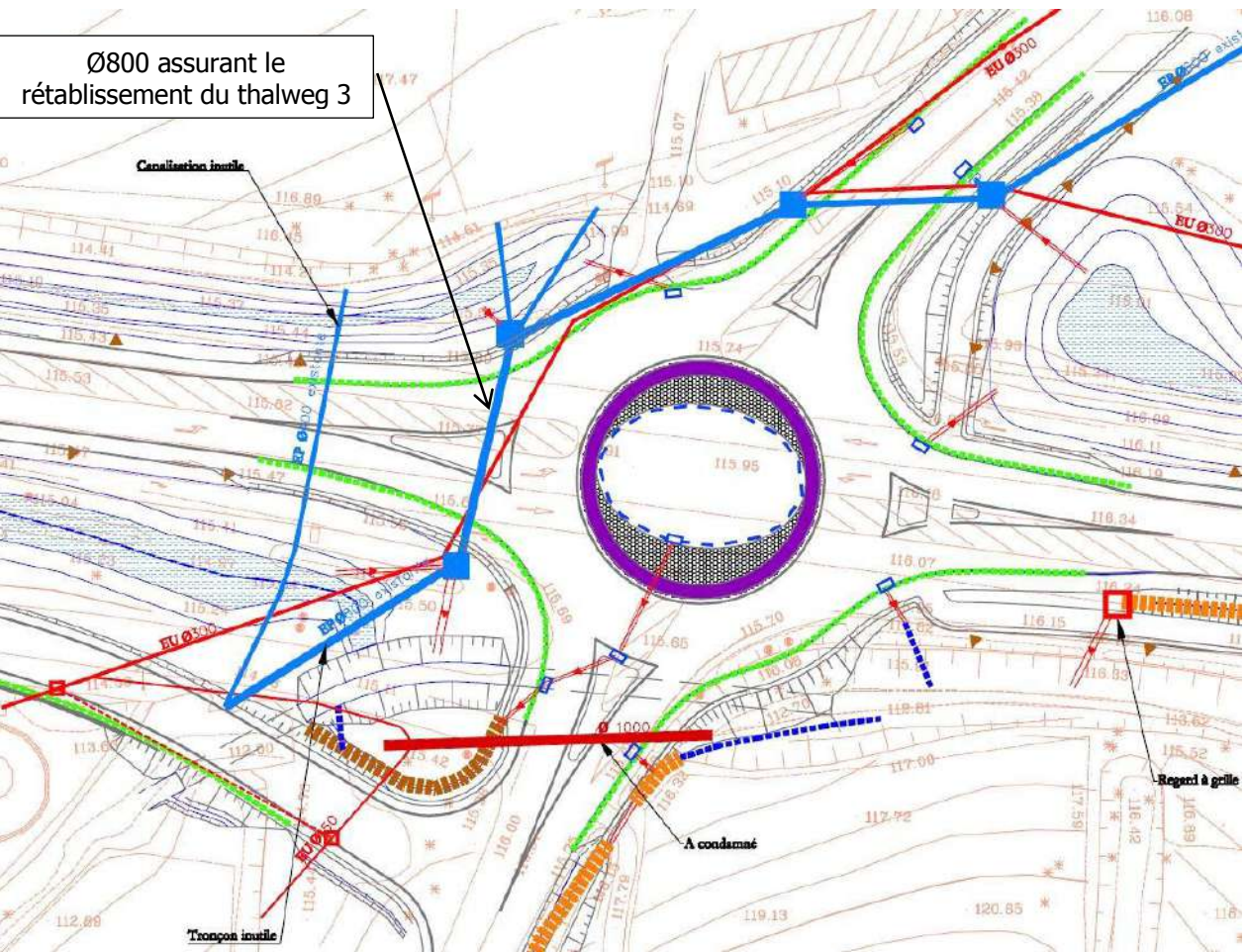
Figure 10 : Extrait du plan DCE du giratoire RN164/RD1 au droit du thalweg 3
