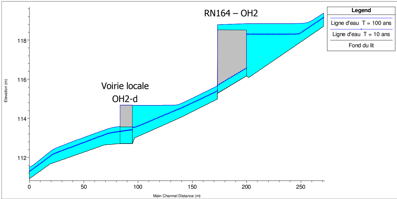
Figure 6 : Thalweg 2 - Lignes d'eau au droit de l'ouvrage - Etat initial
