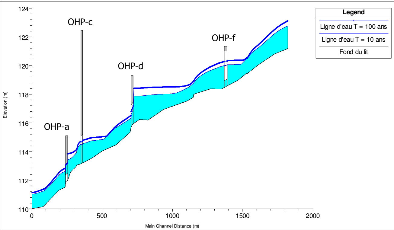
Figure 29 : Le ruisseau de Plémet- Lignes d'eau - Etat projet
