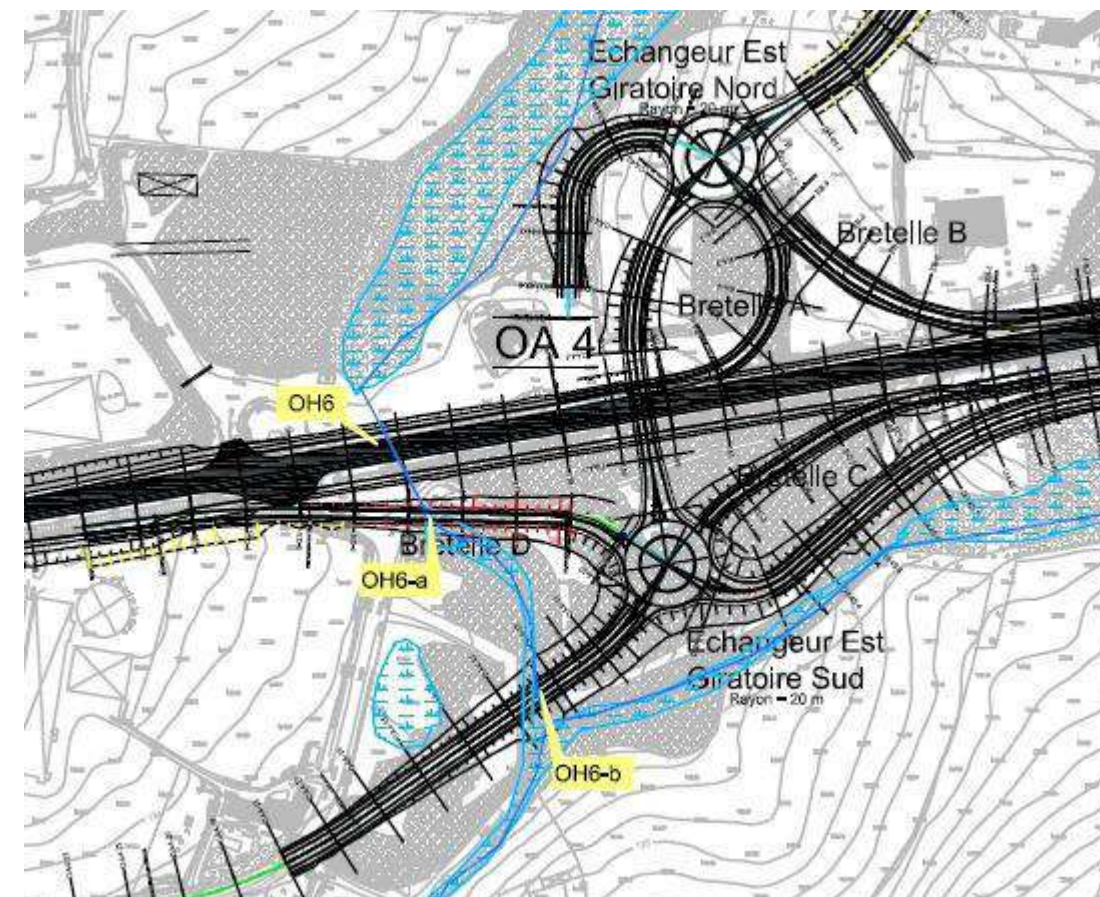
Figure 17 : Thalweg 6 - situation après aménagement
