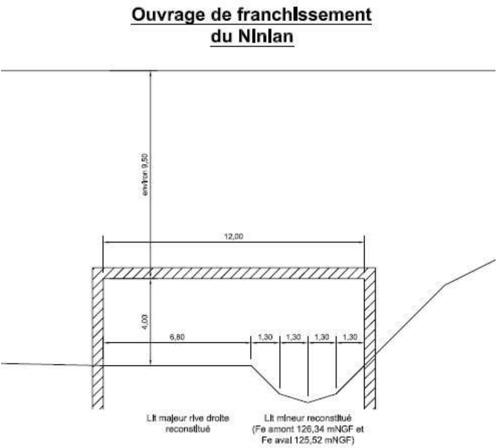
Figure 24 : Le Ninlan - Ouvrage OH8 projet
