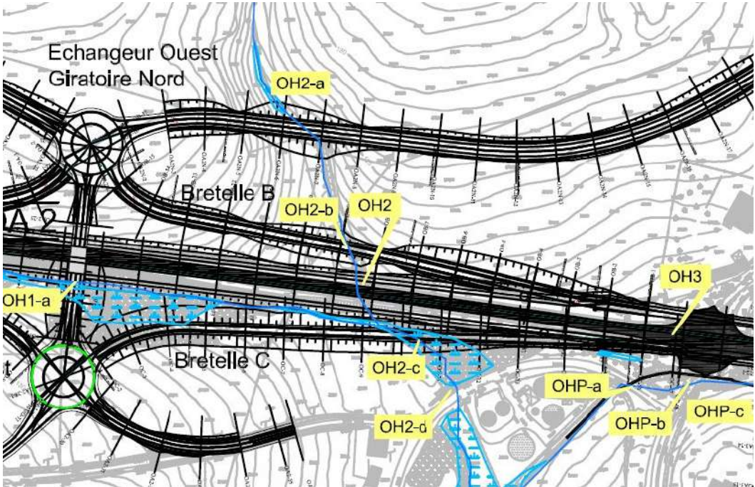
Figure 7 : Thalweg 2 - situation après aménagement
