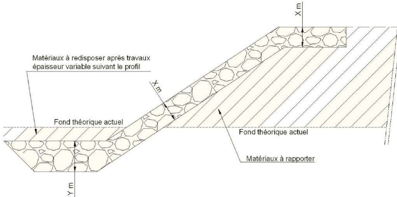
Figure 30 : Coupe de principe d'enrochement de fond de lit et de berges d'un cours d'eau
