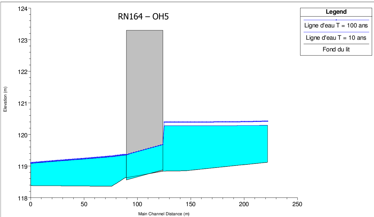
Figure 13 : Thalweg 5- Lignes d'eau au droit de l'ouvrage - Etat initial
