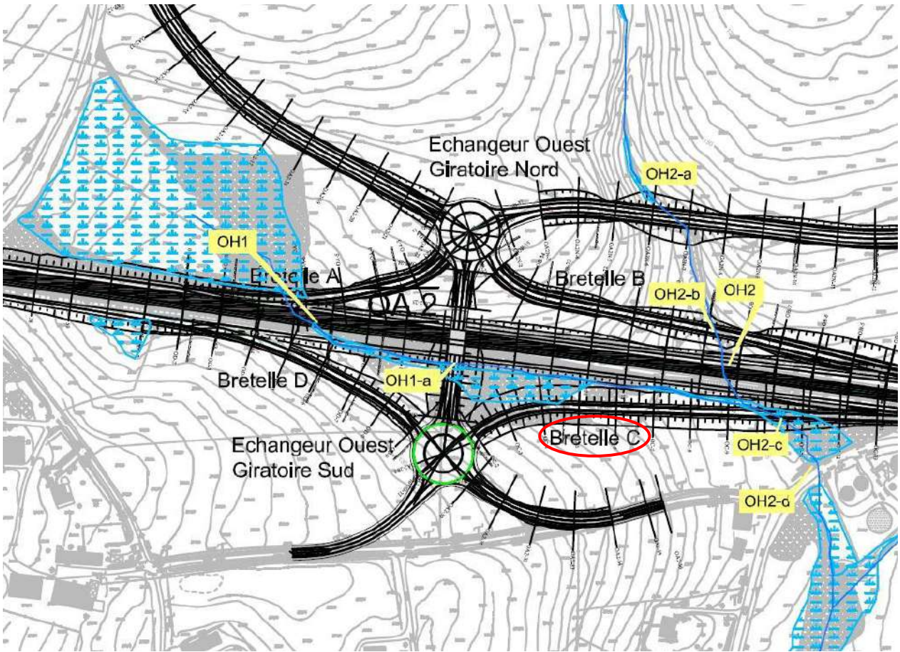
Figure 3 : Thalweg 1 - situation après aménagement
