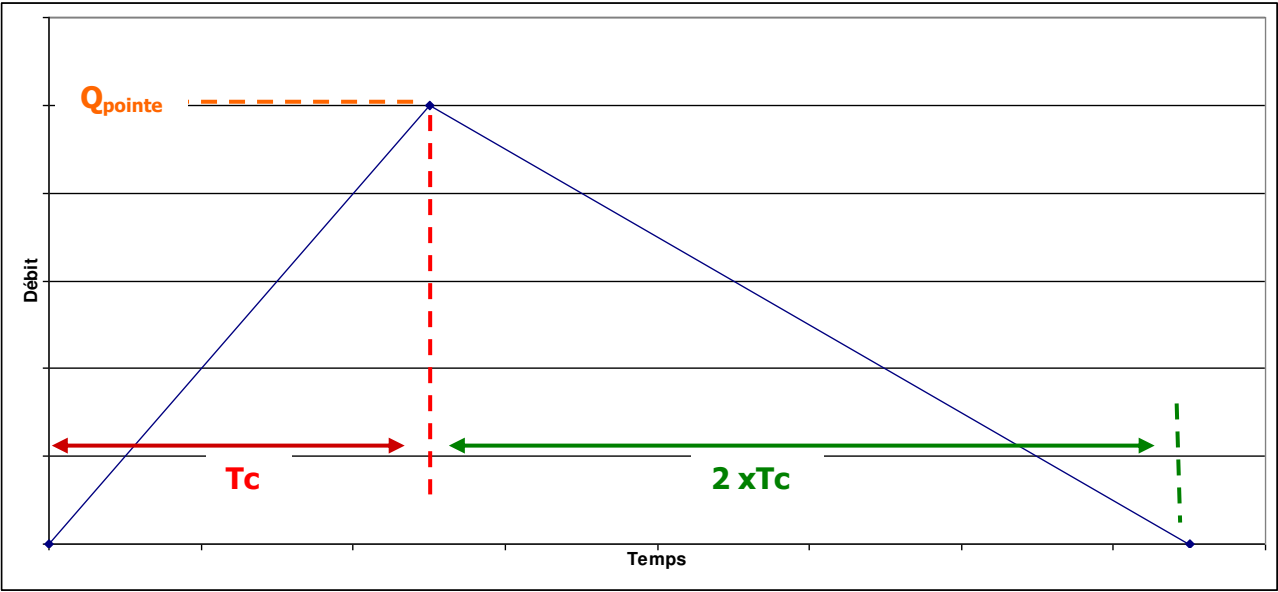
Figure 1 : Hydrogramme triangulaire type
