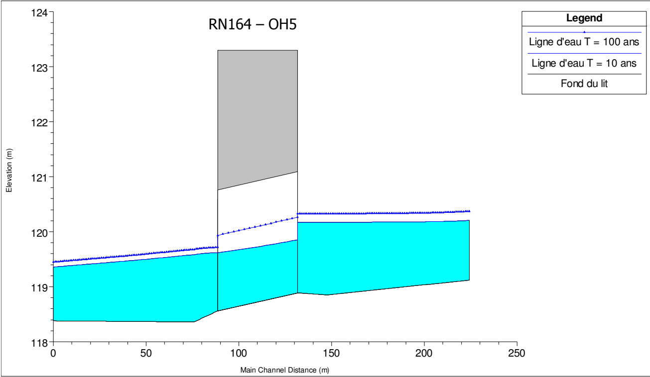
Figure 15 : Thalweg 5 - Lignes d'eau au droit de l'ouvrage - Etat projet
