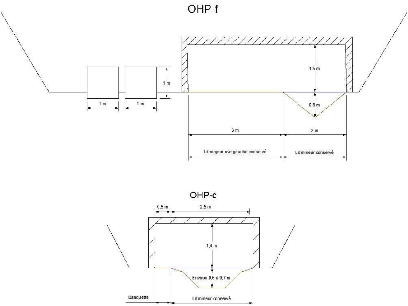
Figure 28 : Plémet - Ouvrages projet
