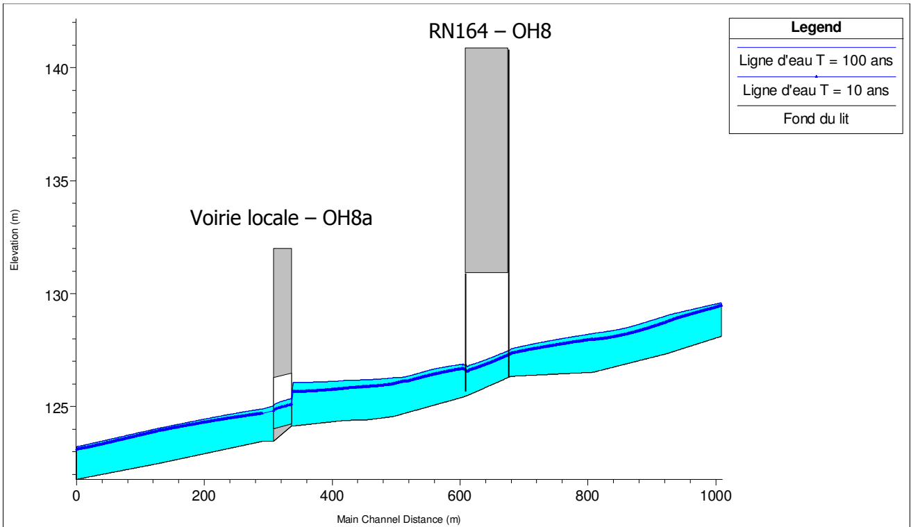
Figure 25 : Le Ninlan- Lignes d'eau au droit de l'ouvrage - Etat projet
