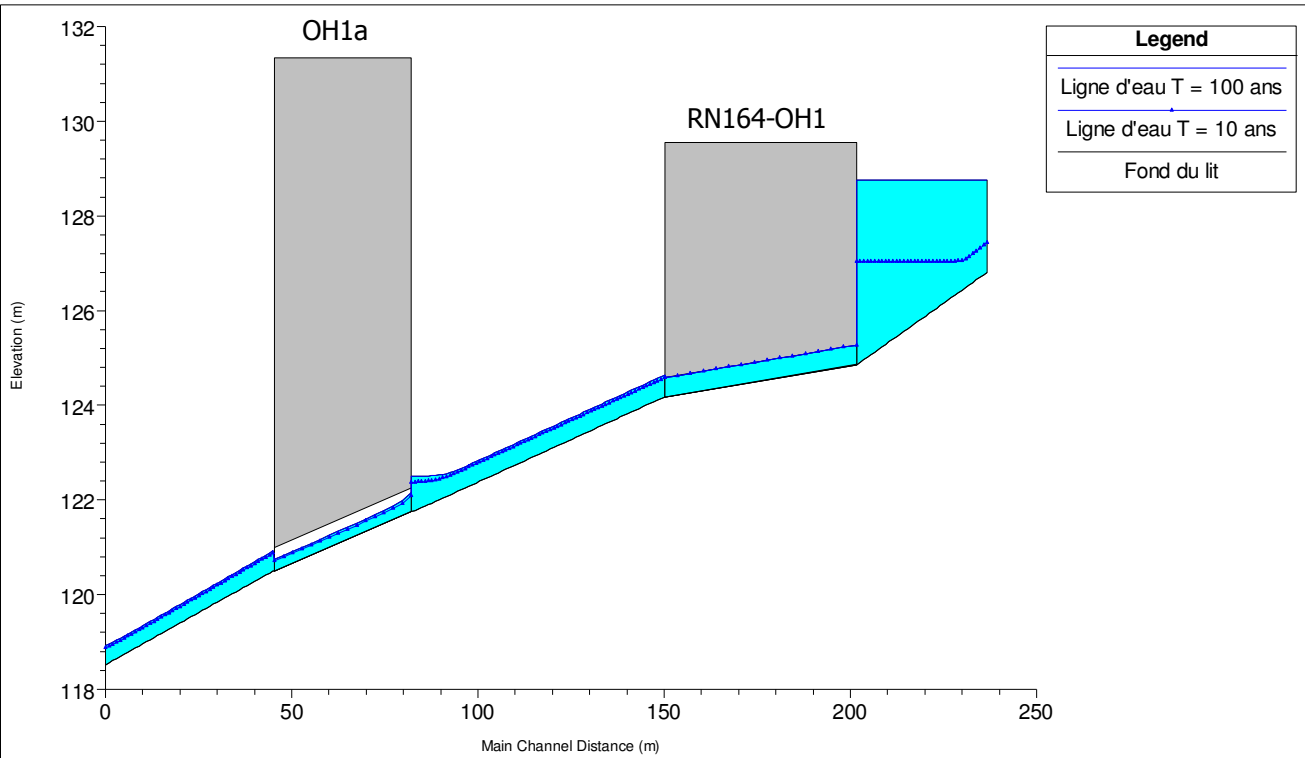
Figure 5 : Thalweg 1 : Lignes d'eau au droit de l'ouvrage - Etat projet
