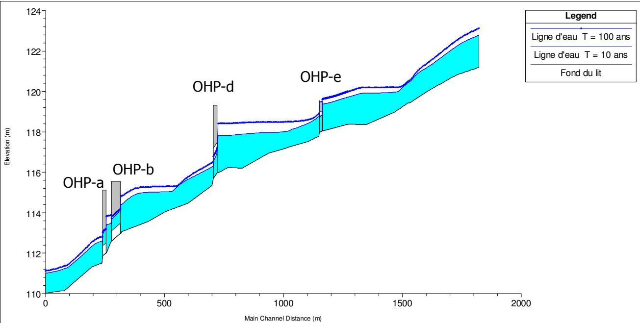
Figure 26 : Le ruisseau de Plémet- Lignes d'eau - Etat initial
