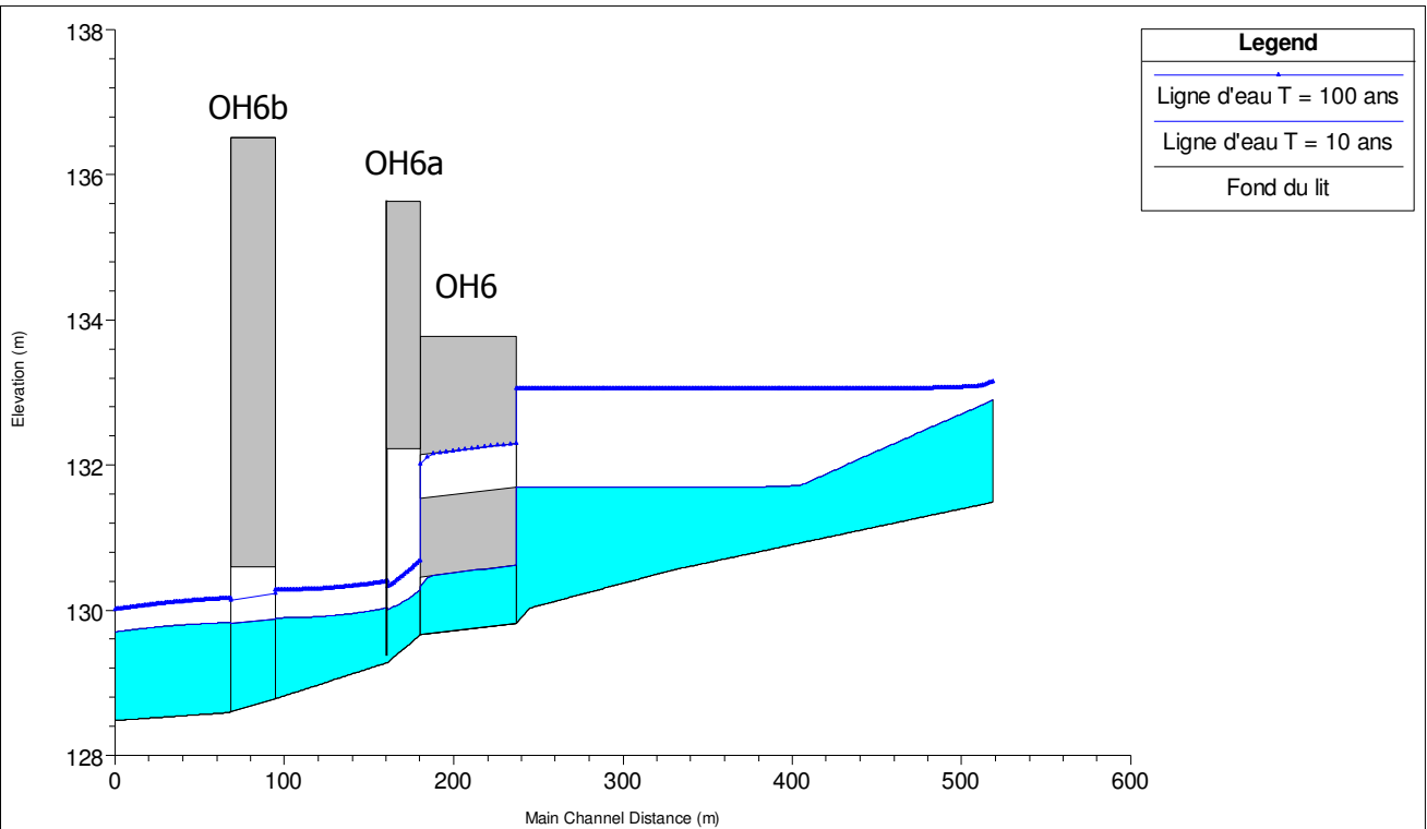
Photographie 21 : Thalweg 6- Lignes d'eau au droit de l'ouvrage - Etat projet.
