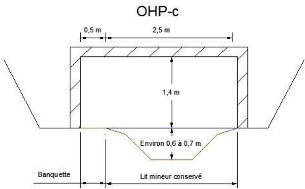
Figure 28 : Plémet - Ouvrages projet
