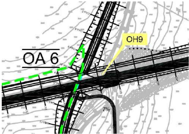
Figure 21 : Thalweg 9 - situation après aménagement
