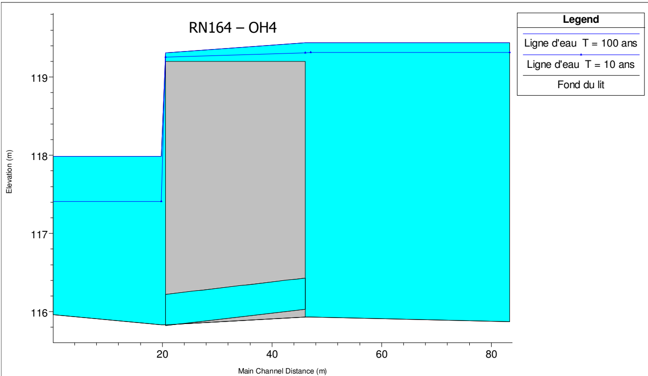
Figure 11 : Thalweg 4- Lignes d'eau au droit de l'ouvrage - Etat initial
