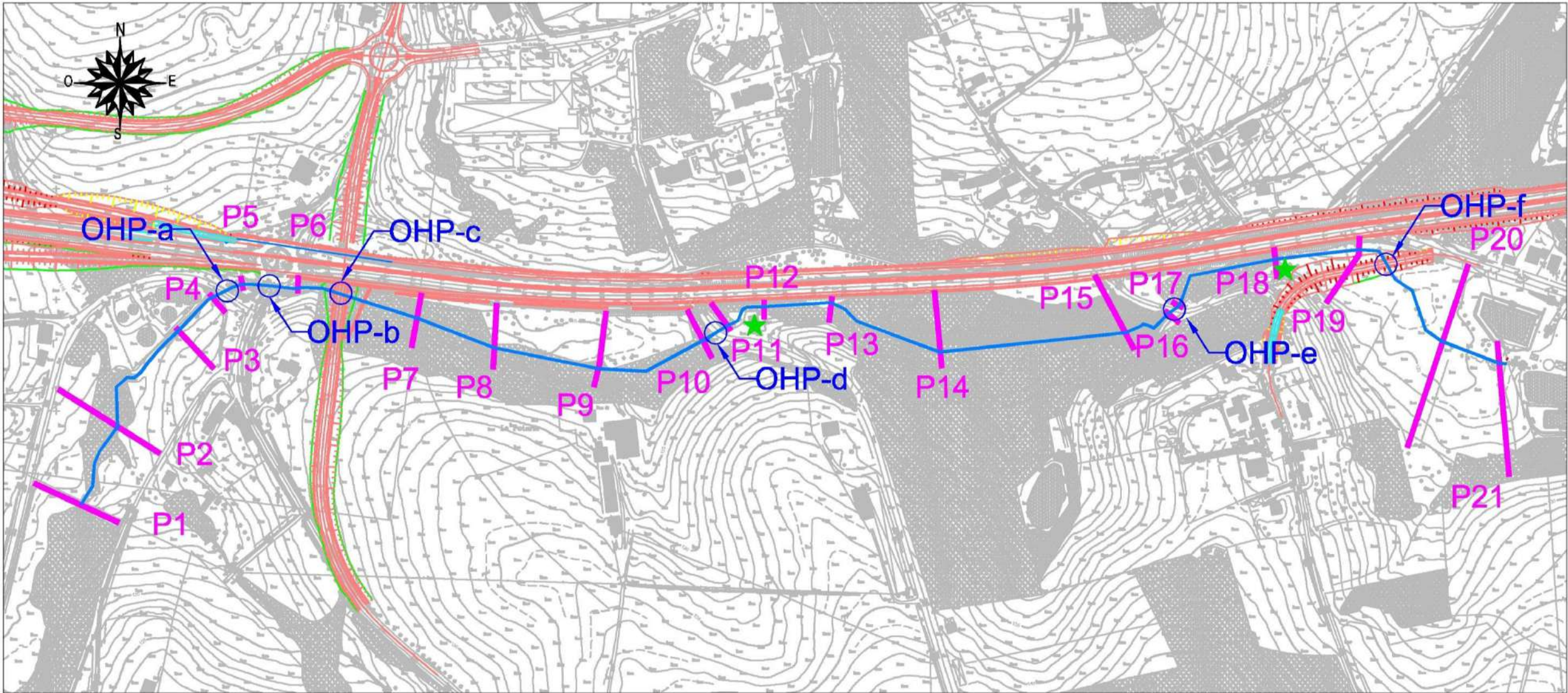
Figure 32 : Plémet- Localisation des profils en travers, ouvrages et enjeux
