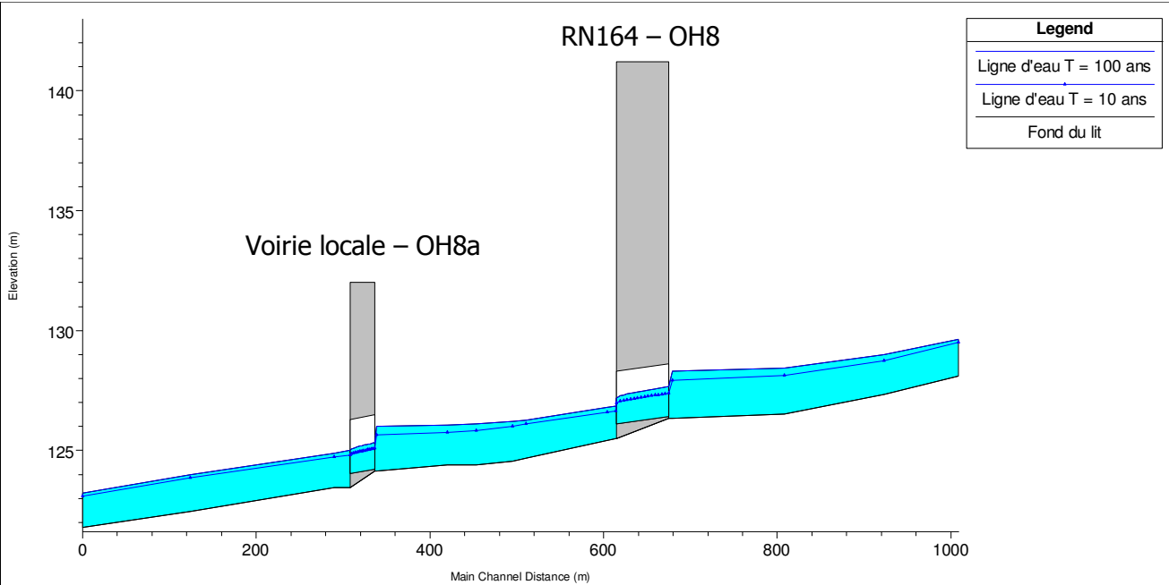
Figure 23 : Le Ninian- Lignes d'eau au droit de l'ouvrage - Etat initial
