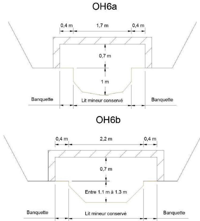
Figure 18 : Thalweg 6 - Ouvrages projet
