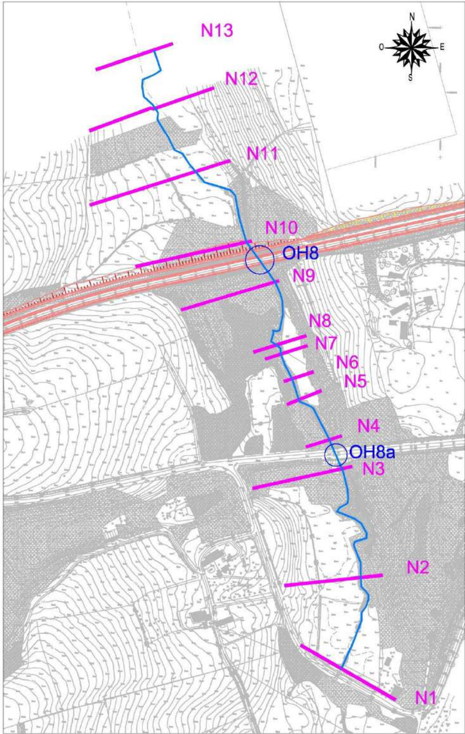
Figure 31 : Ninian - Localisation des profils en travers et ouvrages
