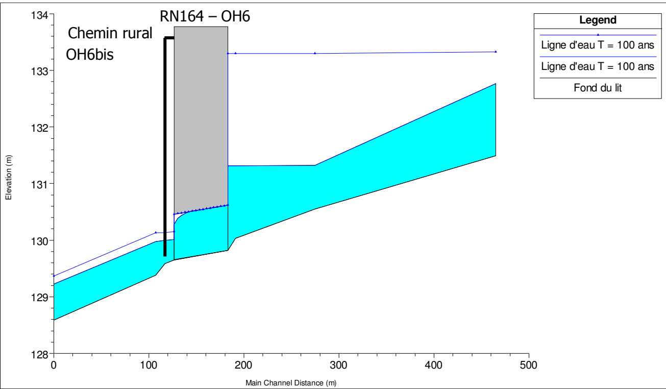
Figure 16 : Thalweg 6- Lignes d'eau au droit de l'ouvrage - Etat initial
