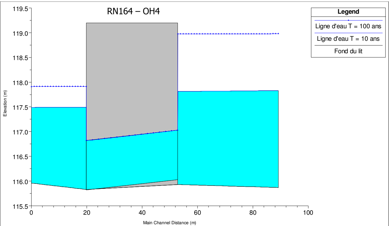
Figure 12 : Thalweg 4- Lignes d'eau au droit de l'ouvrage - Etat projet
