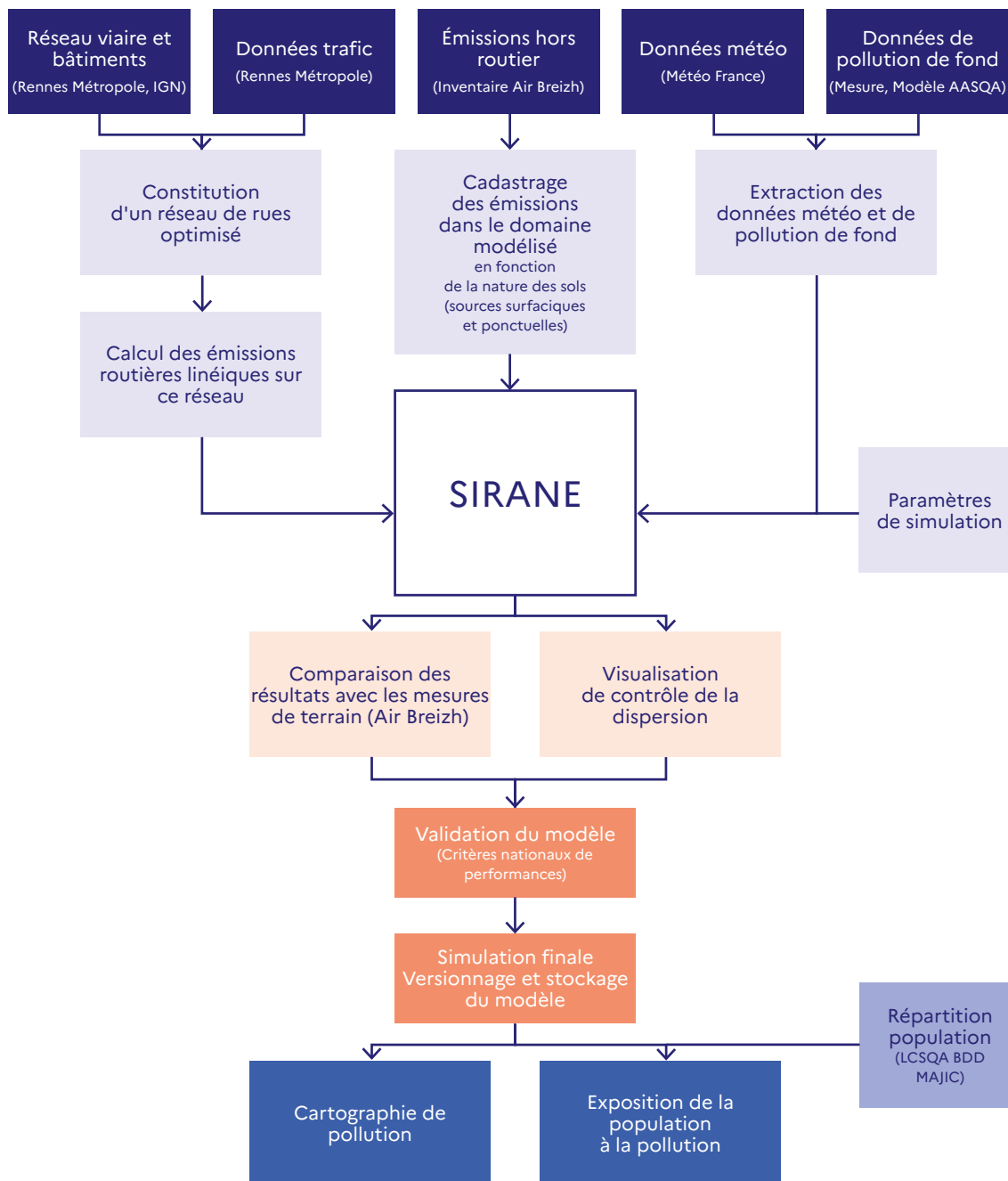
Figure 9 : Vue d'ensemble du processus d'élaboration du modèle urbain de Rennes Métropole
