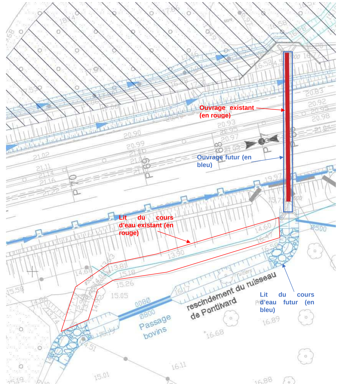
Figure 47 : Rescindement du ruisseau de Pontlivard (source ARCADIS)
