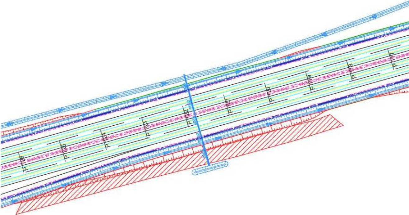
Figure 48 : Rétablissement du Clos de la Rompe (source ARCADIS)
