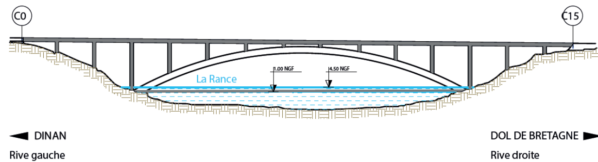
Figure 12 : Schéma d'un nouveau pont arc (source CEREMA)
