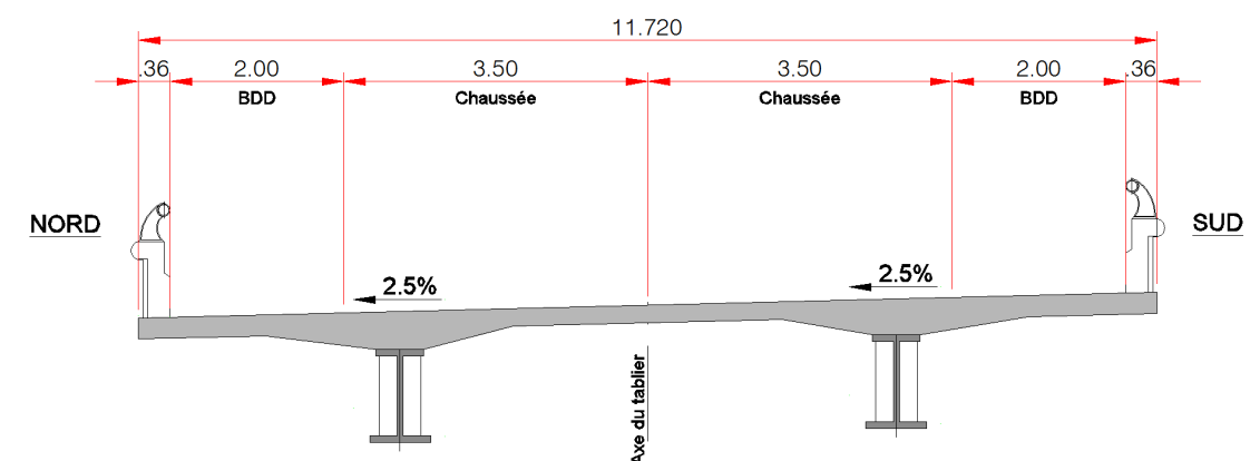
Figure 7 : Coupe de l'ouvrage existant (source CEREMA)
