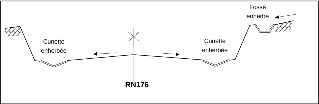
Figure 36 : Profil en travers en déblai et rasant (source ARCADIS)
