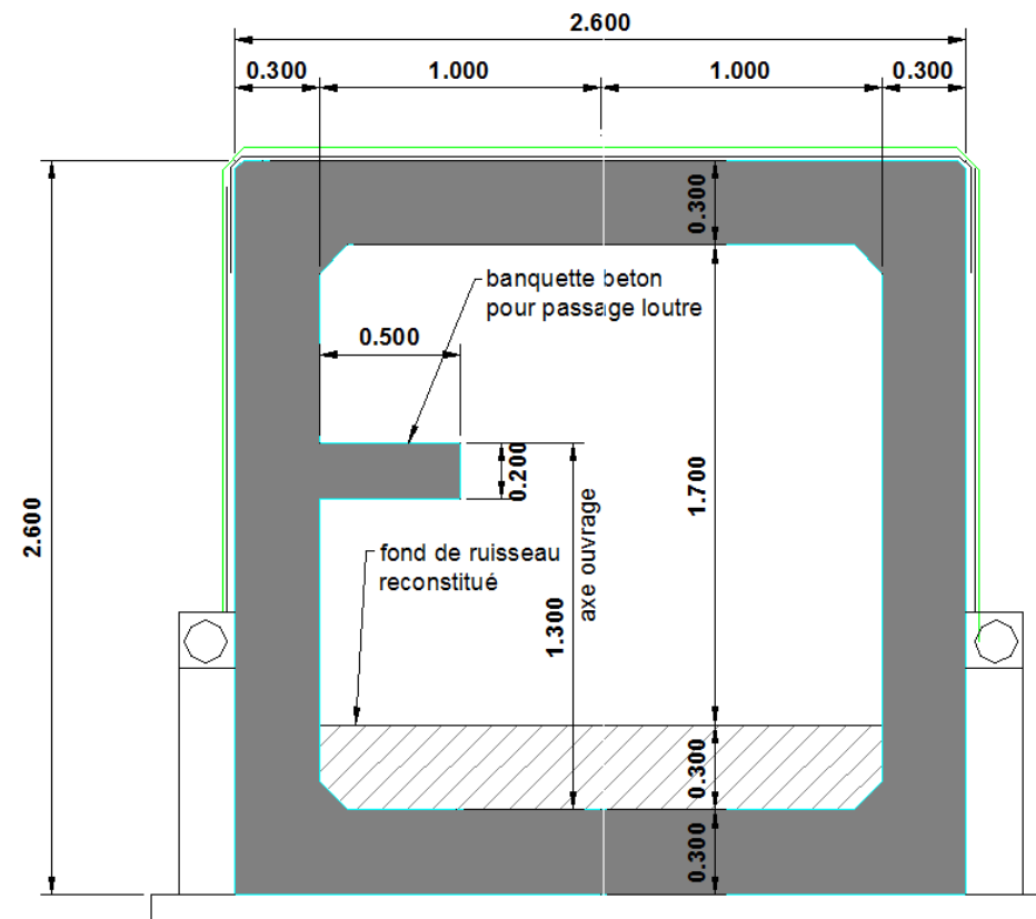
Figure 43 : Coupe transversale de l'OH (source ARCADIS)
