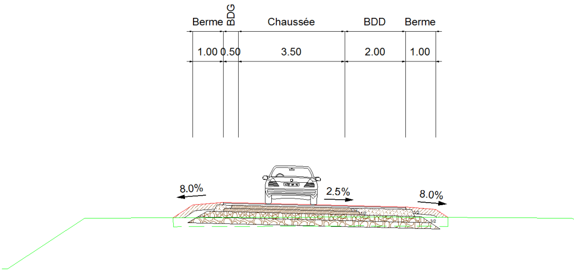
Figure 29 : Profils en travers des bretelles de l'échangeur avec la RD 366 (source ARCADIS)
