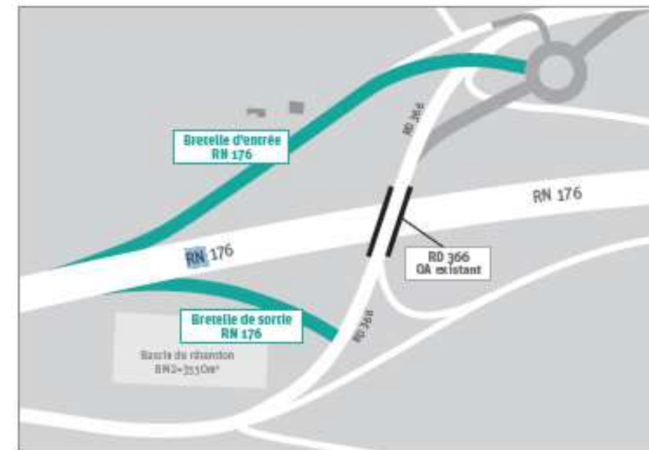
Figure 15 : Schéma de la variante A de l'aménagement de l'échangeur avec la RD366 (source SENNSE)
