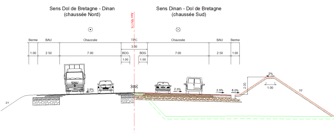
Figure 25 : Profil en travers de la section courante en remblai avec merlon (source ARCADIS)
