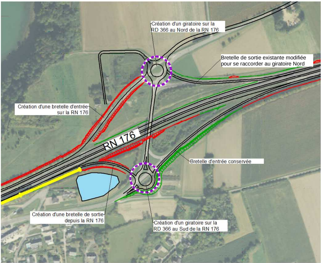
Figure 28 : Echangeur avec la RD 366 (source ARCADIS – fond de plan IGN)
