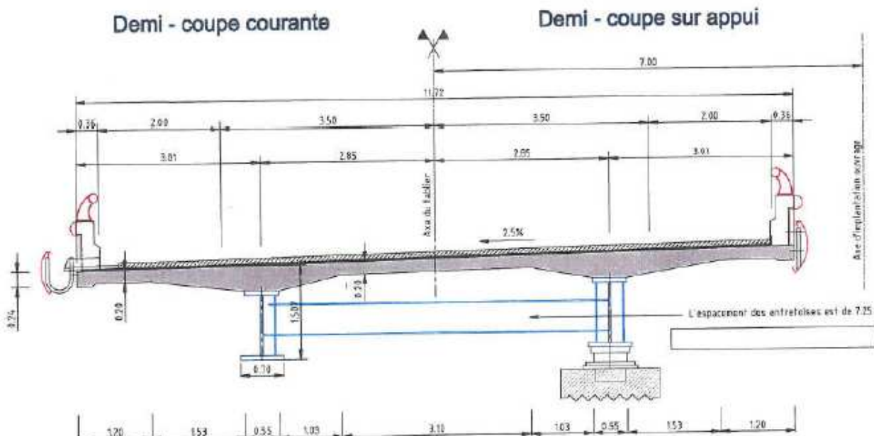
Figure 32 : Coupe transversale du tablier actuel (source EPOA 1999 – SETRA)
