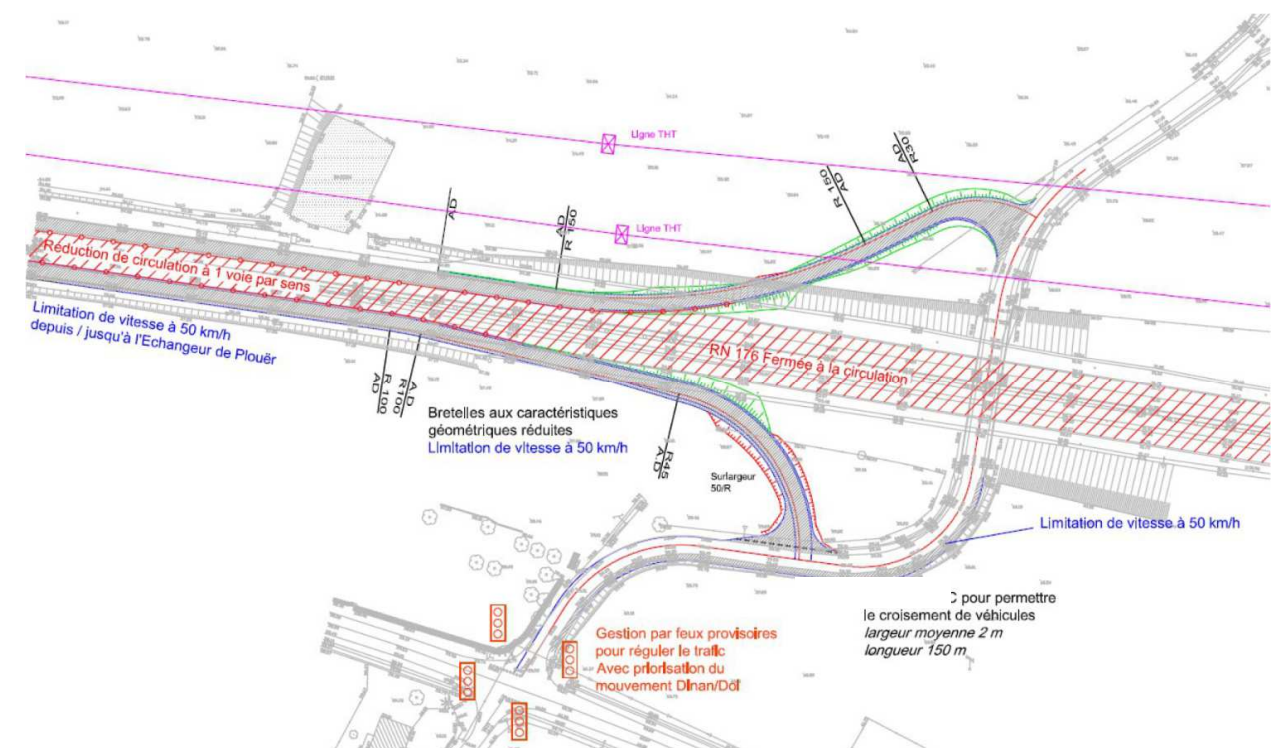
Figure 52 : Bretelles provisoires au droit de la VC de la Boissanne (source ARCADIS)
