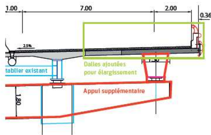
Figure 10 : Schéma des appuis supplémentaires (source CEREMA)
