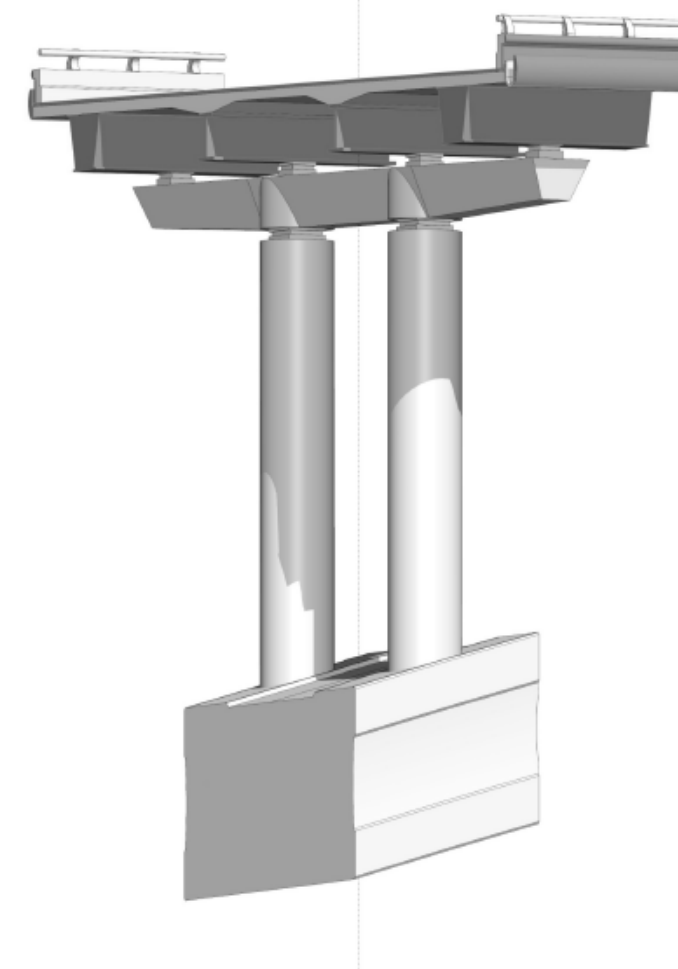
AXONOMETRIE DE LA PILE
