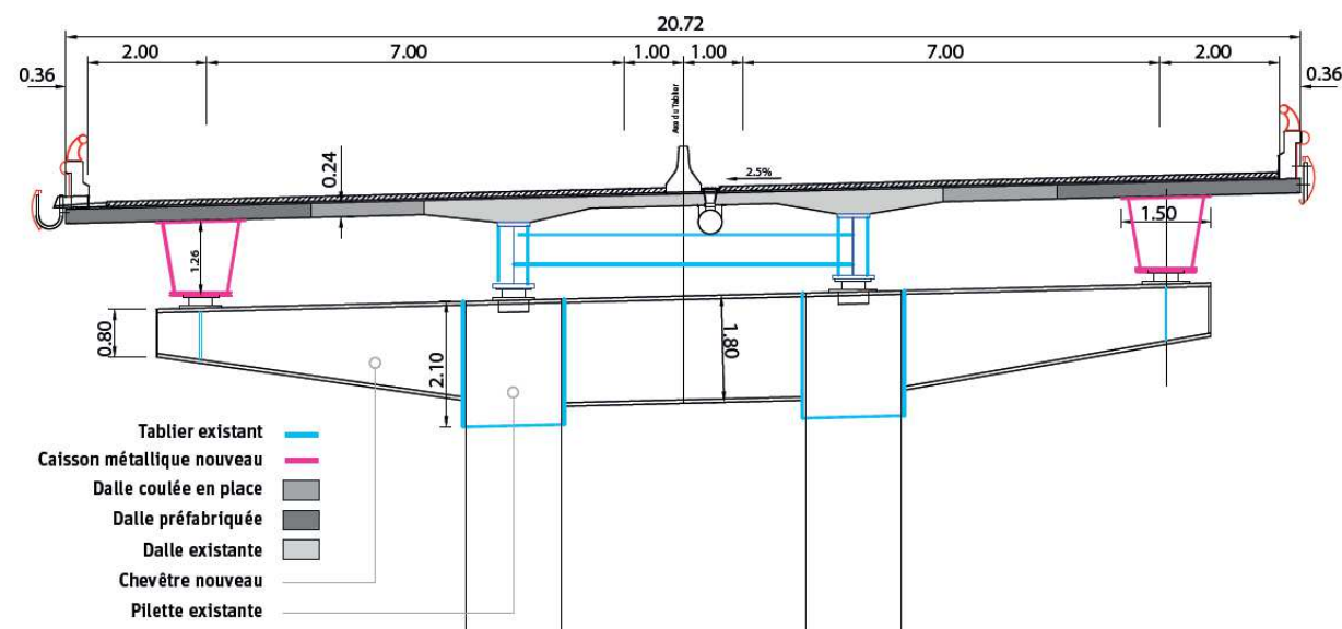
Figure 11 : Variante 2 – Coupe sur ouvrage (source CEREMA)
