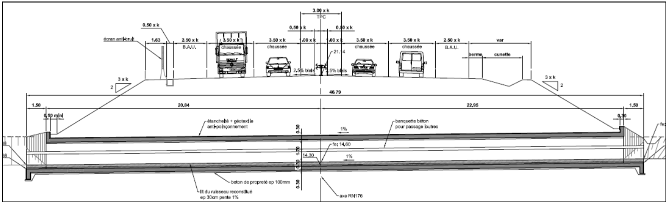
Figure 42 : Coupe longitudinale de l'OH (source ARCADIS)
