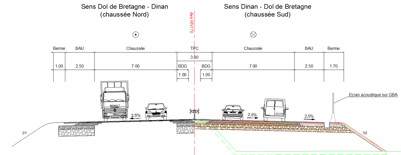
Figure 24 : Profil en travers de la section courante en remblai avec écran acoustique (source ARCADIS)
