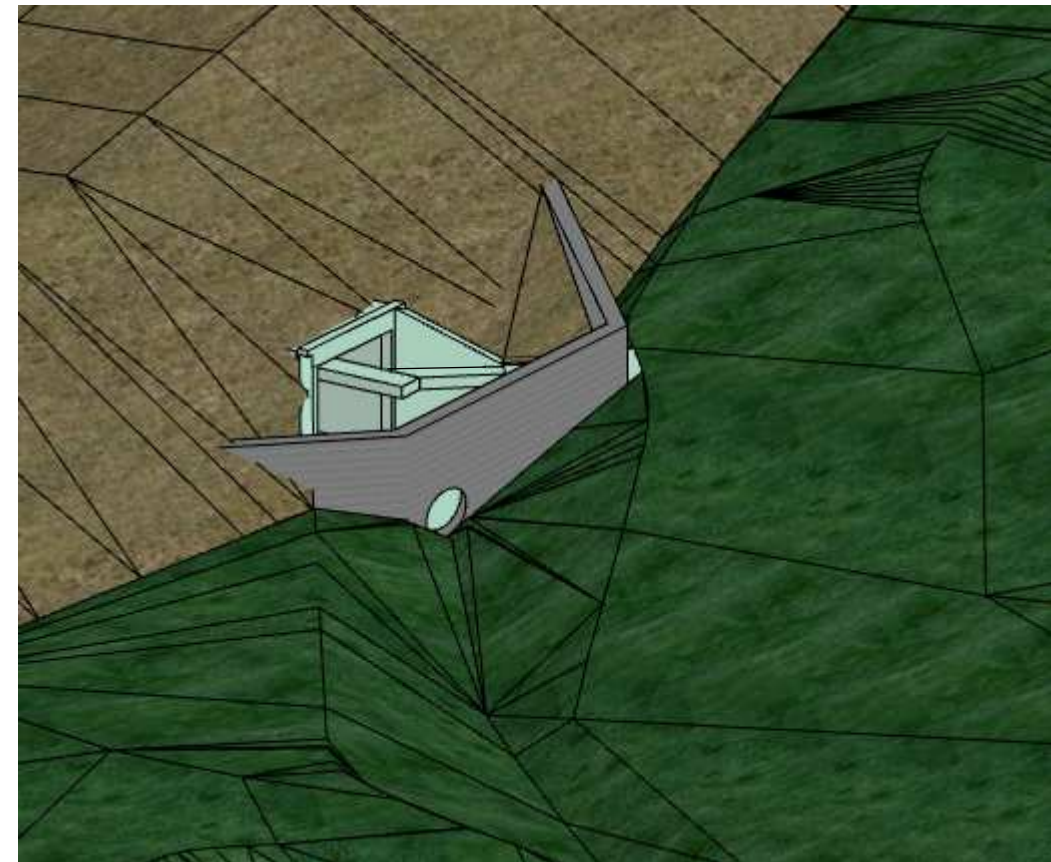
Figure 44 : Représentation de l'ouvrage en 3D en amont de la RN176 (source ARCADIS)
