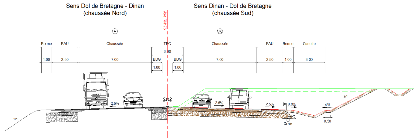
Figure 23 : Profil en travers de la section courante en déblai (source ARCADIS)
