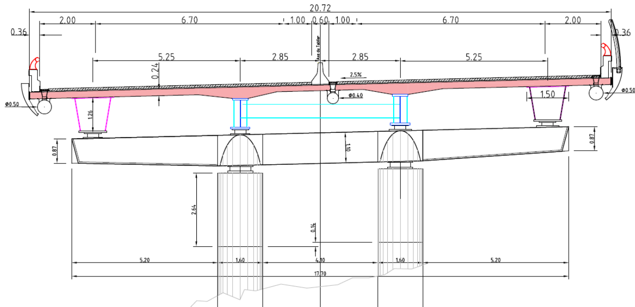
Figure 33 : Profil en travers de l'élargissement du pont Chateaubriand (source CEREMA)
