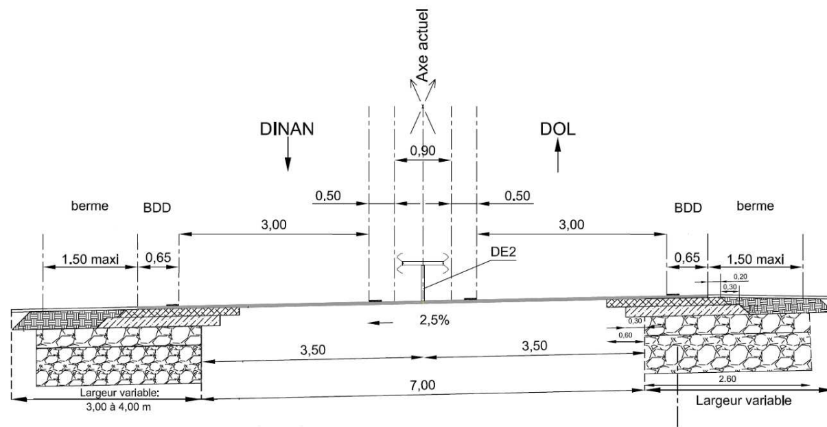
Figure 6 : Profil en travers actuel (source DIR Ouest)
