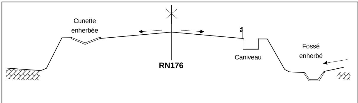
Figure 37 : Profil en travers en remblai (source ARCADIS)
