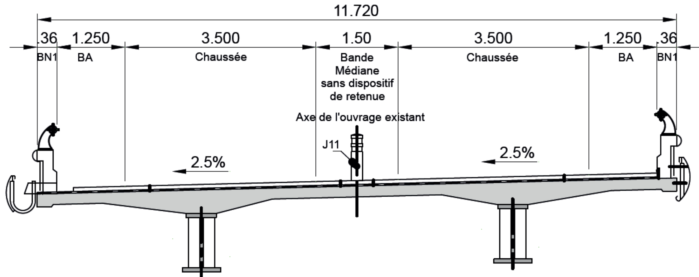
Figure 9 : Variante 1 – Coupe sur ouvrage (source CEREMA)
