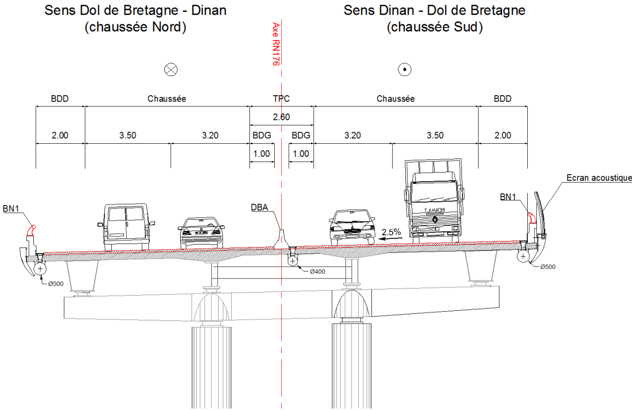
Figure 26 : Profil en travers du Pont Chateaubriand (source ARCADIS)
