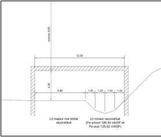
Ouvrage de franchissement du Ninian
