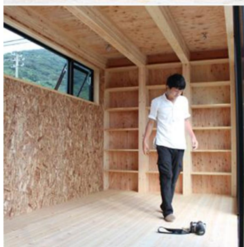
Maison Transportable
