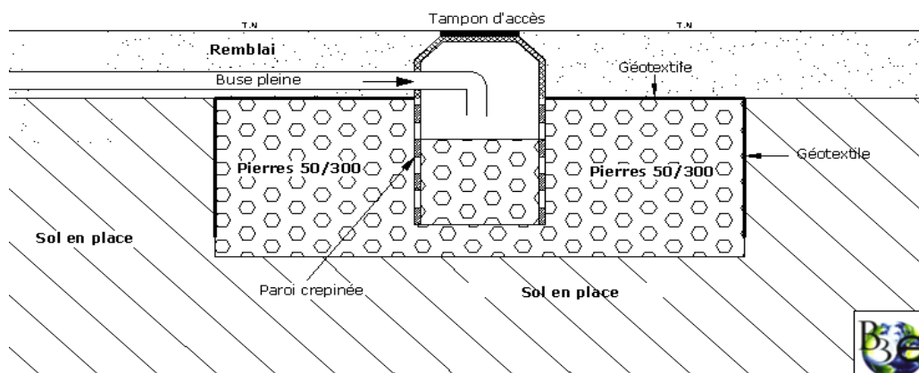
Figure 5 : Coupe schématique d'un puits d'infiltration (source : B3E)
