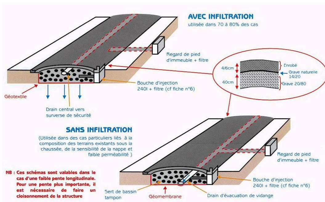
Figure 9 : Schéma de principe des chaussées à structure réservoir
