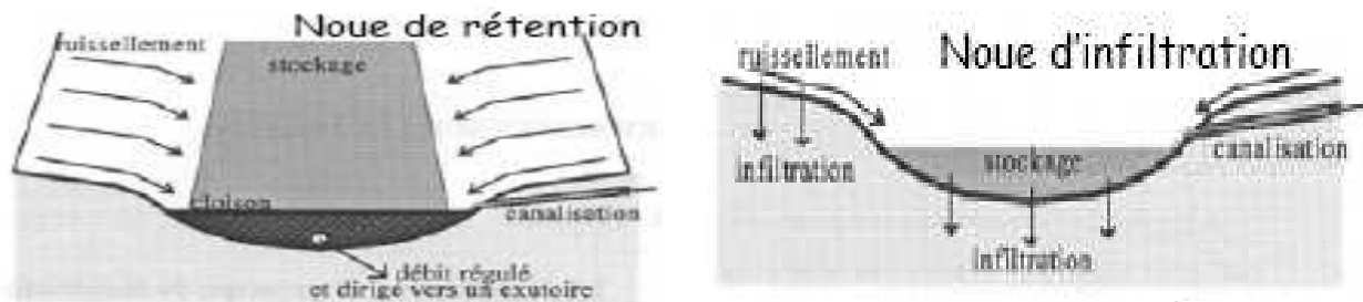
Figure 8 : Schéma de principe d'une noue
