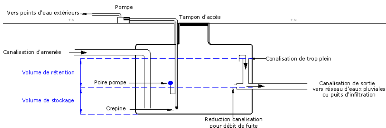
Figure 6 : Schéma d'un réservoir de stockage/ rétention pour les eaux pluviales
