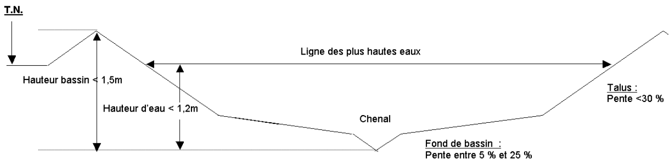
Figure 7 : Coupe schématique d'un bassin de rétention
